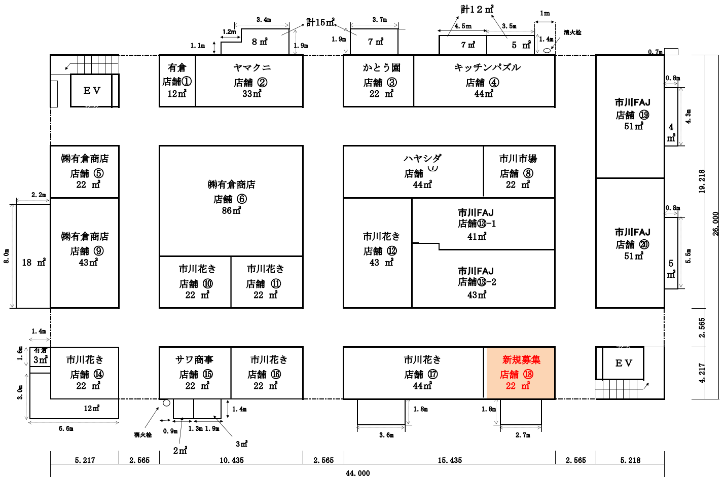
1 階平面図
